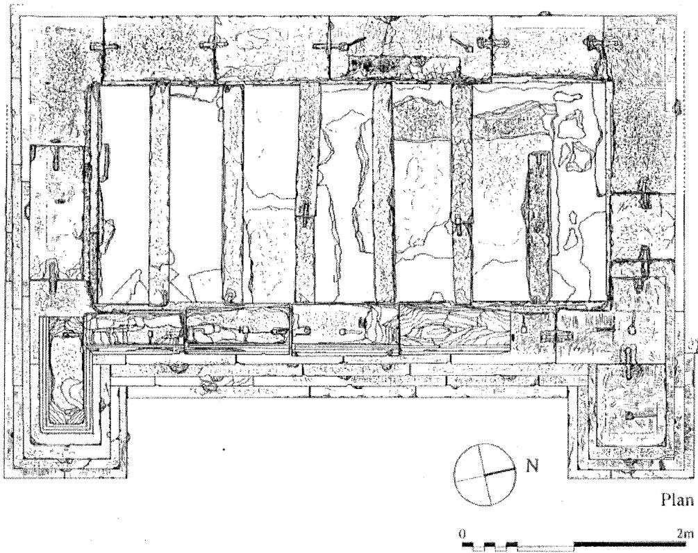
图1 墓廟 | 現状平面図
