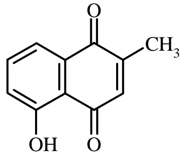
Plumbagin (PLG)
