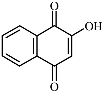
Lawsone (LAS)
