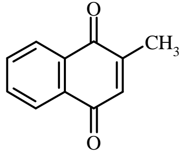
Menadione
