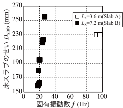
図7 固有振動数
