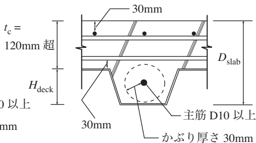
図3 直交異方向性スラブ断面
