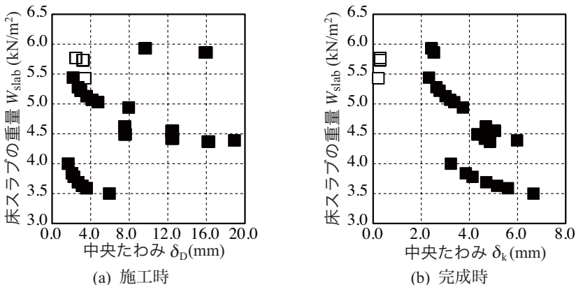
図5 中央たわみ
