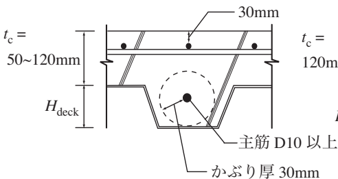
図2 一方向性スラブ断面
