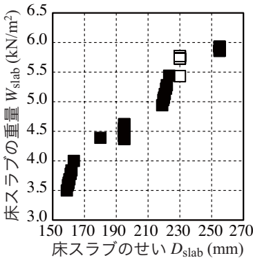
図6 床スラブのせい
