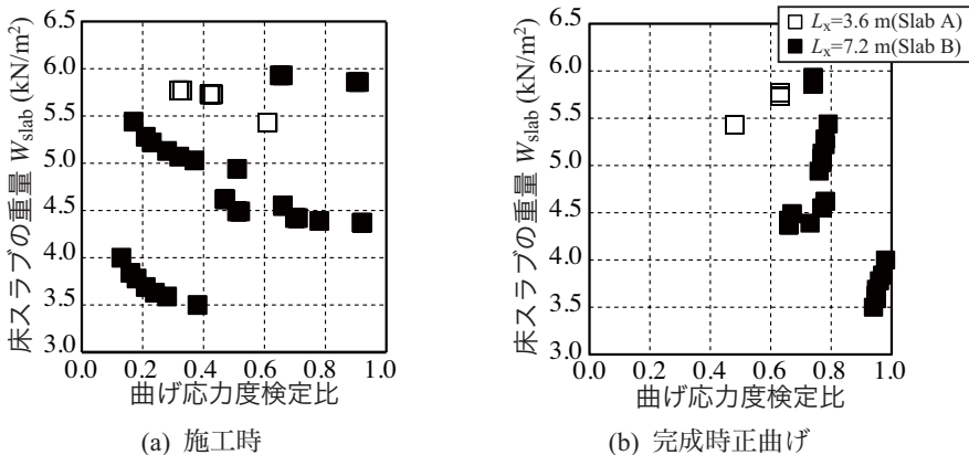
図4 曲げ応力度検定比
