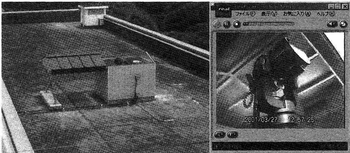
図2：ルーフ開閉式観測室（左）と、望遠鏡（右：ルーフが開いてゆく様子を RealPlayer で観察している）
