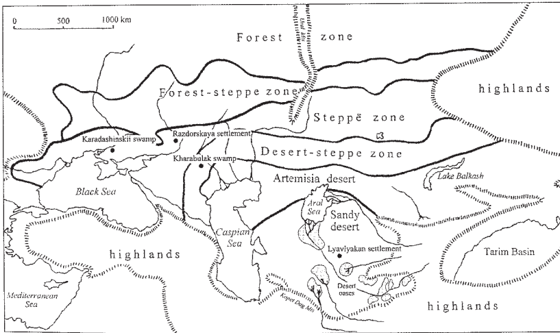
第3図 中央アジアに於ける現在の植生区分図
