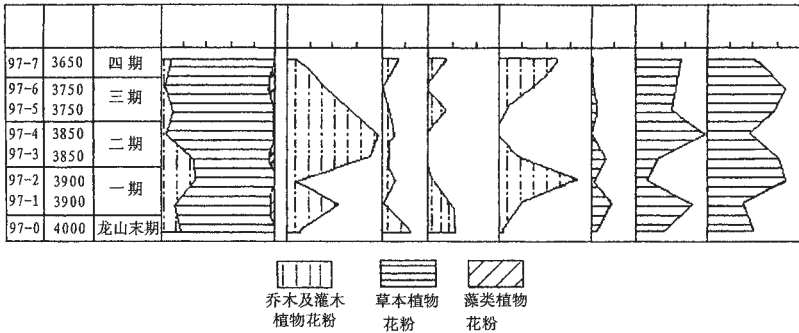
第6図 二里頭遺跡の花粉ダイアグラム (宋豫秦2002年より)
