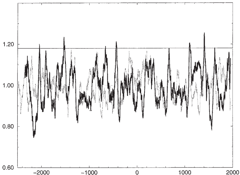
第2図 アメリカでの年輪の年代的变化
