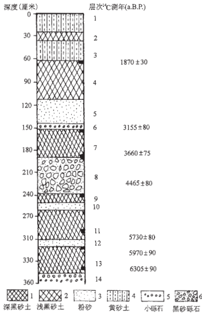
第5図 老虎山遺跡の柱状図と考古学編年表
