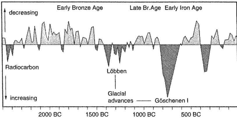
第1図 ヨーロッパにおける炭素14濃度変化と気候変動
