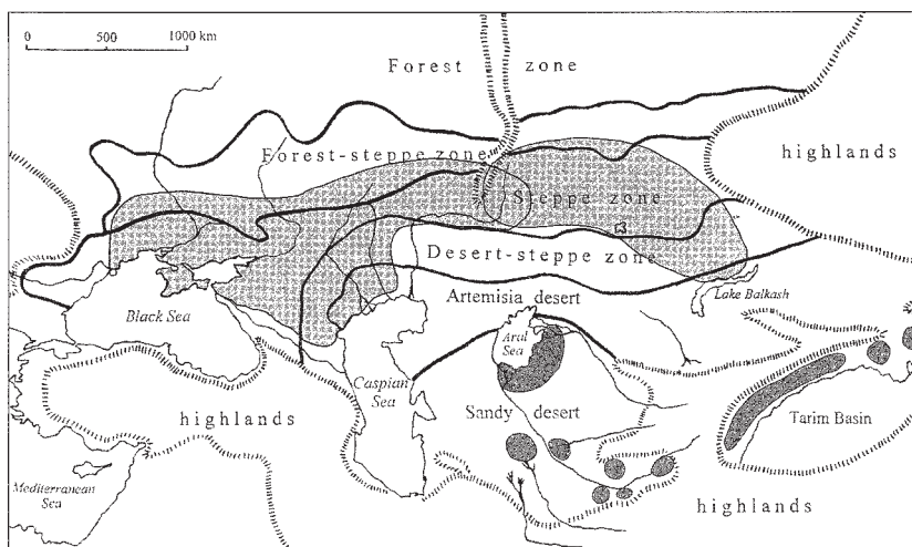
第4図 BC2000-BC1800の中央アジアの植生区分図
