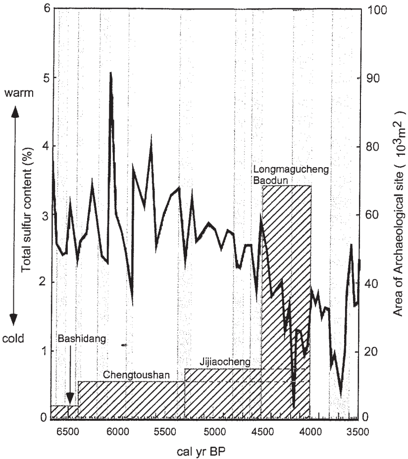
第11図 東郷湖を基準とした環境変化 (Yasuda, et.al., 2004より)
