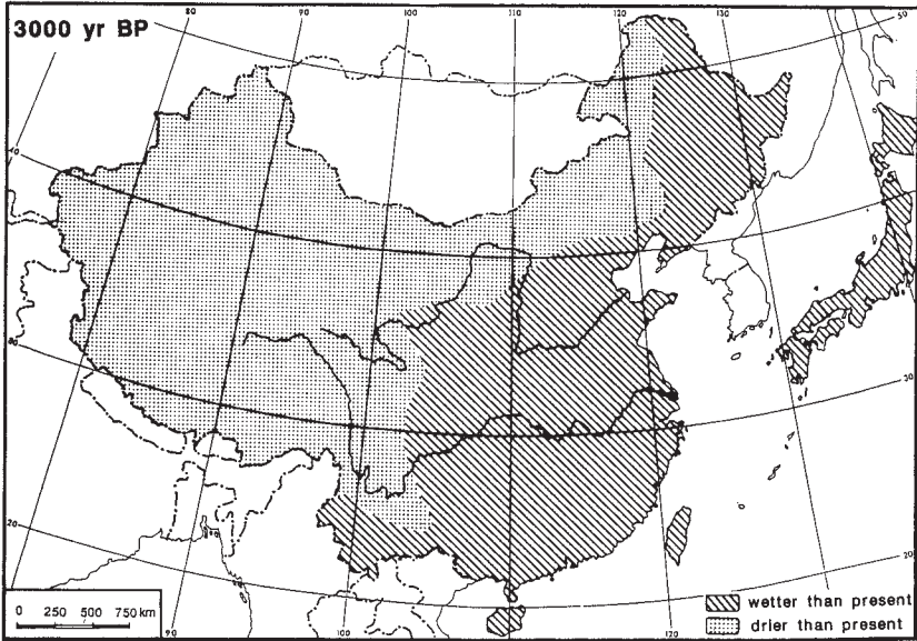
第13図 紀元前1000年頃の乾湿地域図
