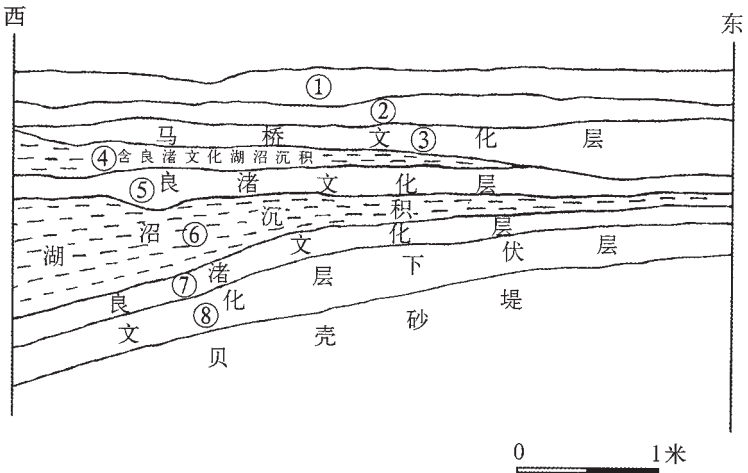
第7図 上海地域の砂堤と馬橋遺跡層序 (周昆叔2007年より)
