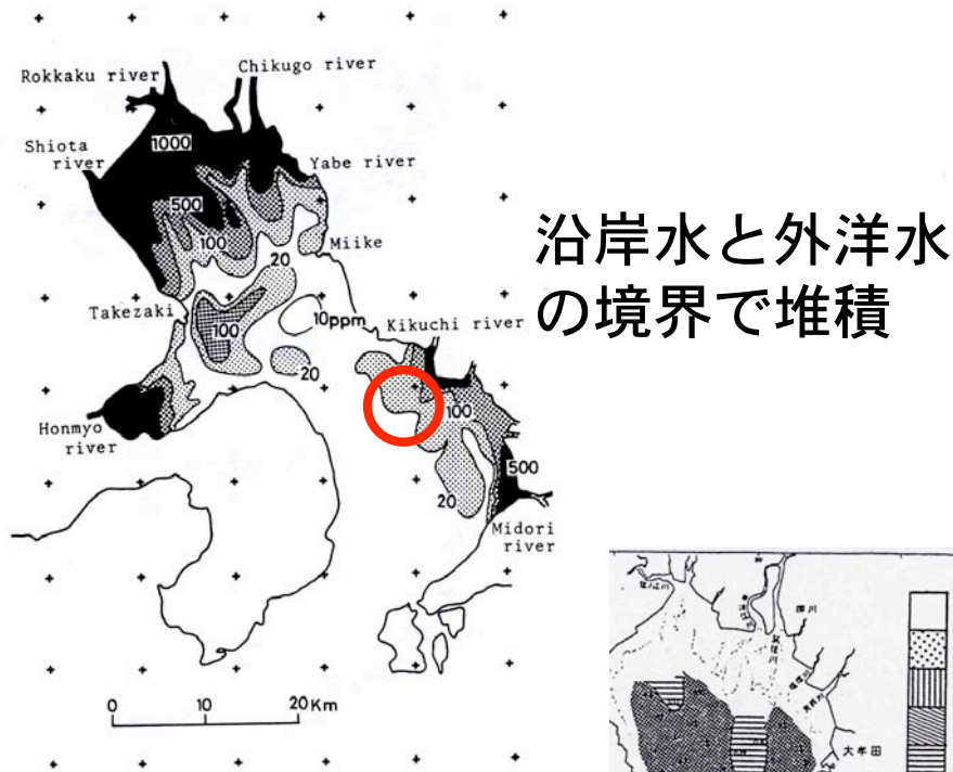
第7図 有明海における浮泥の濃度分布 20) 人工衛星 LANDSAT (1979年12月20日) の写真解 析と船上調査から作図
