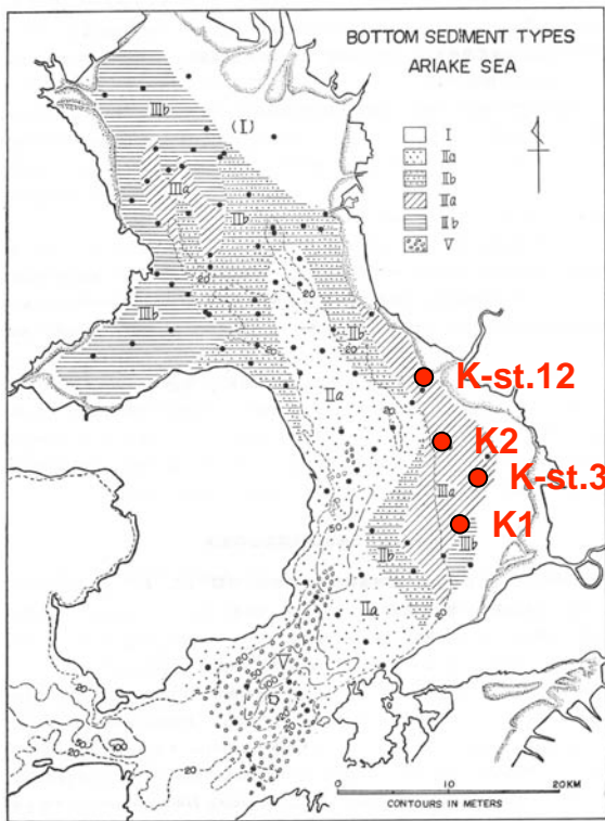
第7図 有明海における堆積型の分布
