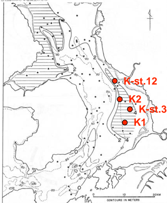
第7図 有明海における堆積型の分布
