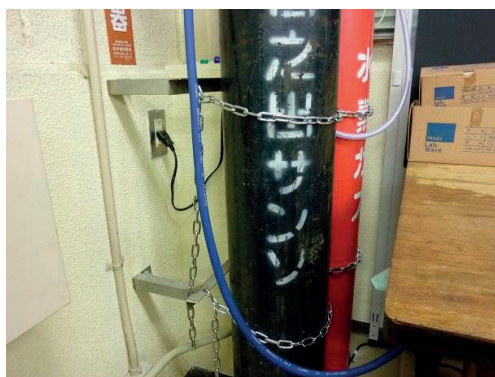
写真 - 8 ボンベ固定支持具
