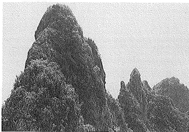
天狗岩 (根子岳山綾をつくる安山岩岩脈: 東方より望む)
