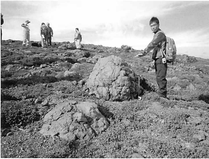
浅間火山 1783 年吾妻火砕流堆積物に含まれるキャベツ状本質岩塊 (2012 年 10 月 13 日 宮縁育夫 撮影).
