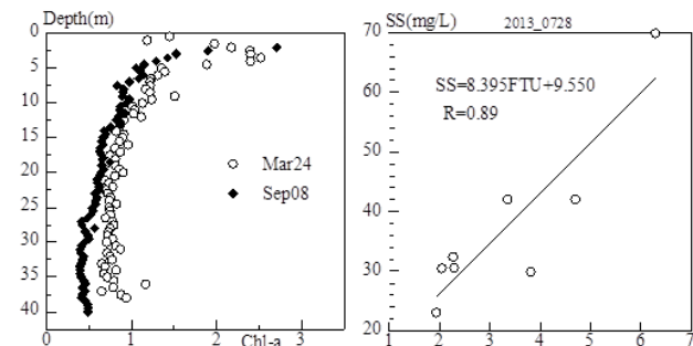
図-8 Chl-a の鉛直分布
