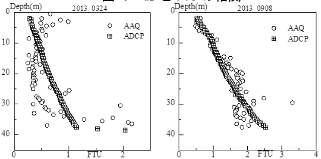
図-7 FTU 鉛直プロファイルの比較
