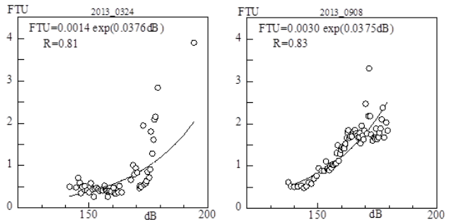
図-6 dB と FTU の相関
