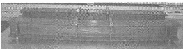
写真1 鋼はり試験体(H-100x100x6x8) (2011年度)
