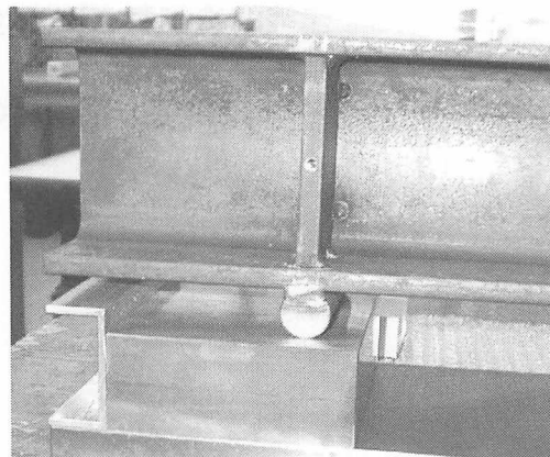
写真3 試験体の左端部の支持状態 (2011年度)
