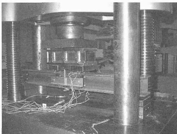
写真2 鋼はりの弾塑性曲げ実験 (全景) (2013年度)
